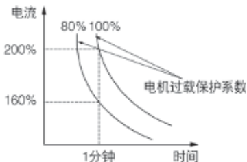
图 FA-1 电机过载保护曲线
