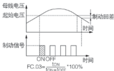
图 FC-1 能耗制动示意图
