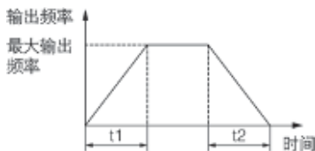
图 F0- 2 加速时间和减速时间示意图
