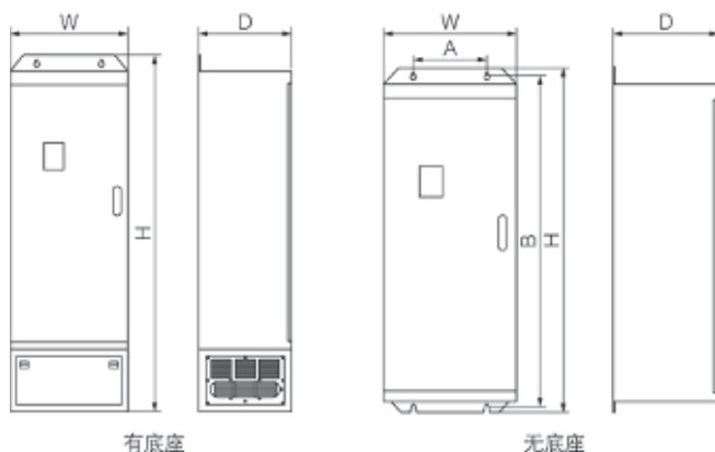
图A-3 160~350kW机型外形尺寸(380V)
