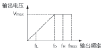
图 F0- 1 电压与频率示意图
