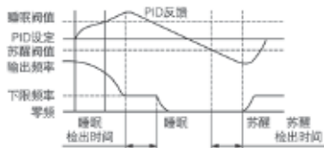
图 F8- 5 第一种睡眠模式示意图
