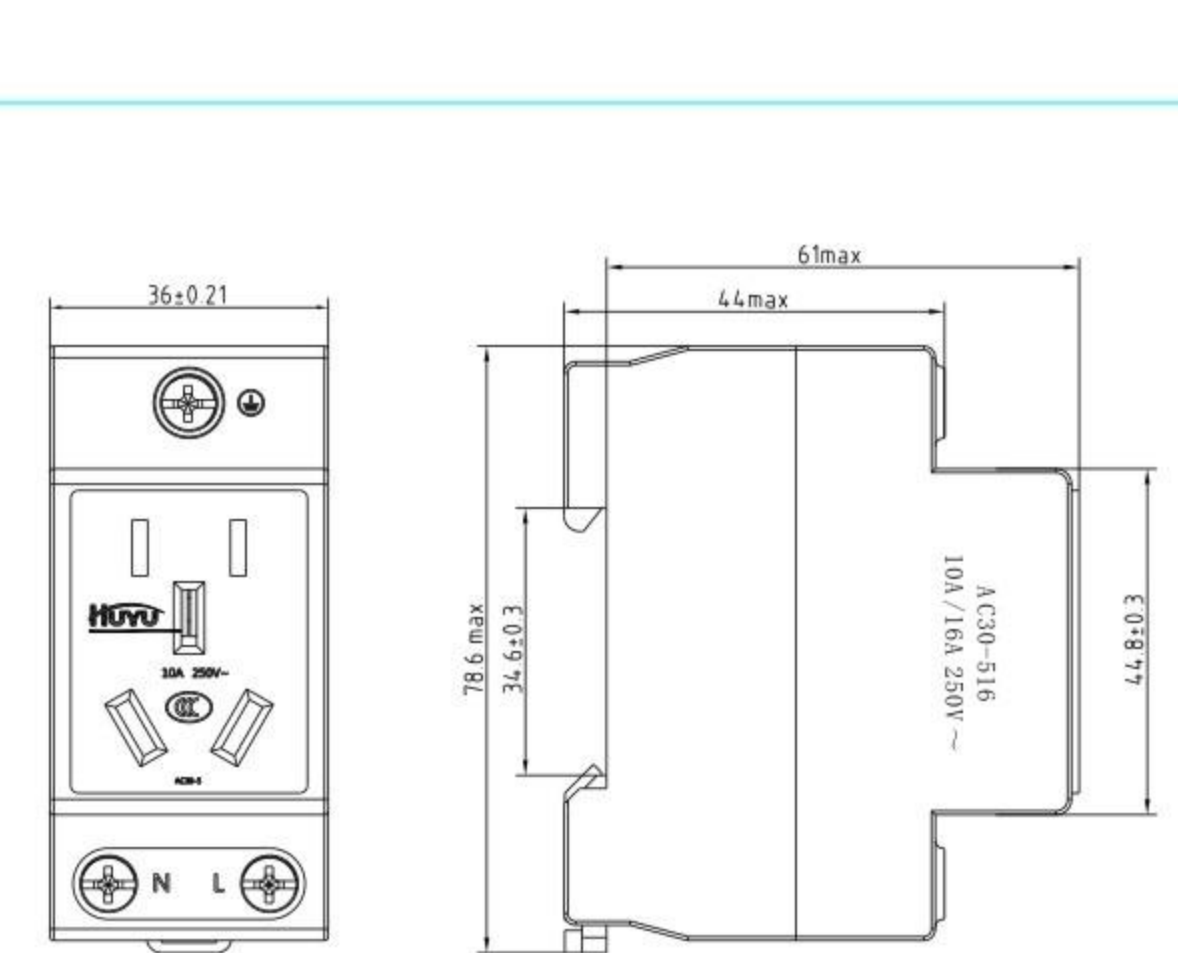
图4 AC30-25/3D 440~外形尺寸及安装尺寸
