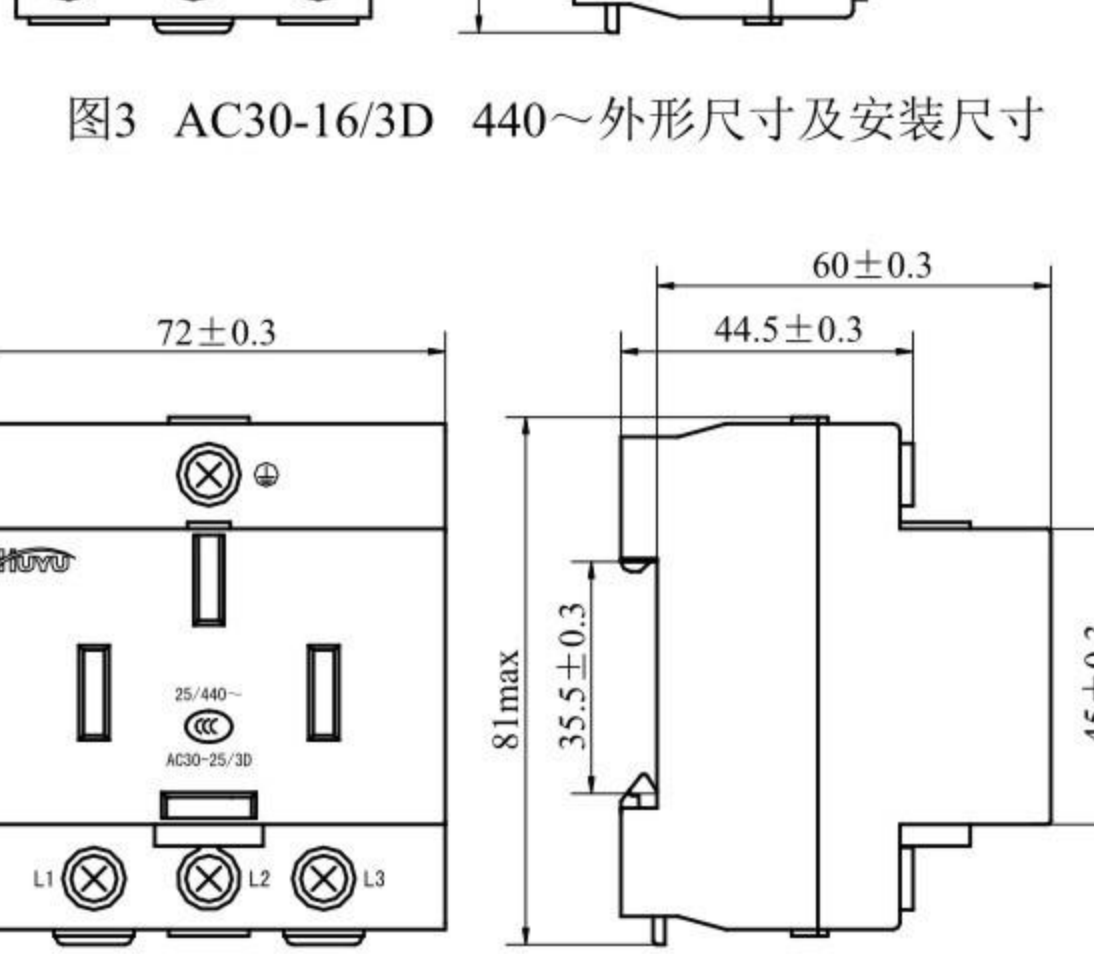
图3 AC30-16/3D 440~外形尺寸及安装尺寸
